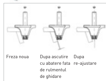
Ghidaj reglabil pe rulmenti axiali cu bile pe bazinul frezei
